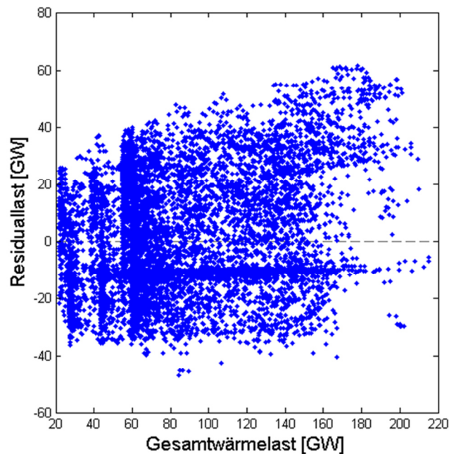
Abbildung 37: Zusammenhang zwischen simulierter Residual- und Wärmelast
