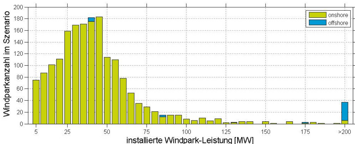
Abbildung 14: Größe der Windparks im Szenario
