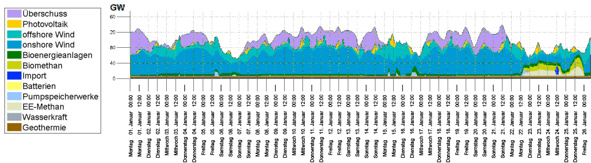
Abbildung 19: Windreiche Januarwochen
