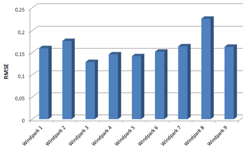
Abbildung 85: RMSE der Prognose für alle Parks
