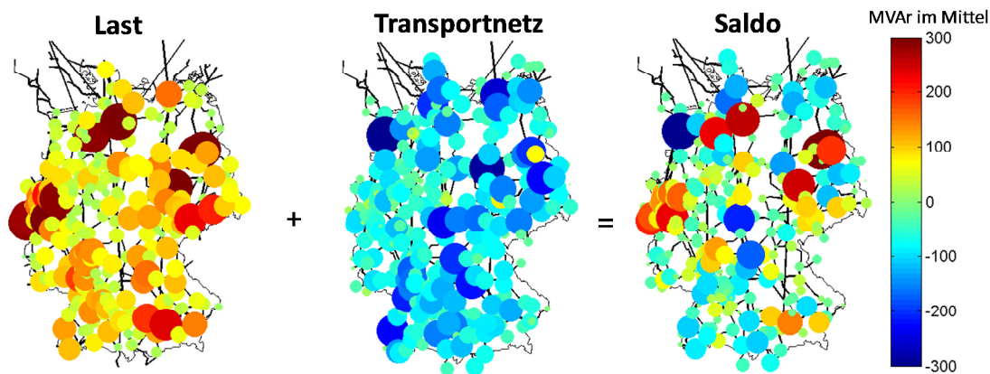
Abbildung 108: Simulierter durchschnittlicher Blindleistungsbedarf der Lasten und des HöS-Netzes im 100%-EE-Szenario, sowie die Bilanz. Positive Blindleistung bedeutet einen induktiven Blindleistungsbezug, negative Blindleistung einen kapazitiven.
