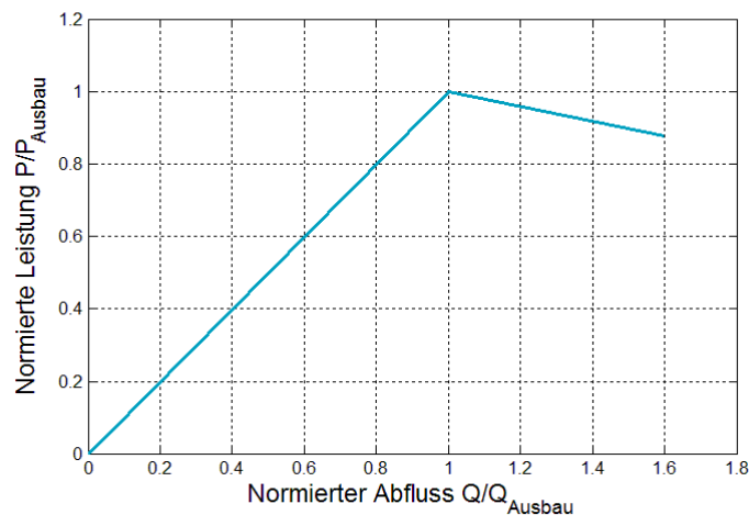
Abbildung 39: Verwendete Wasserkraftkennlinie
