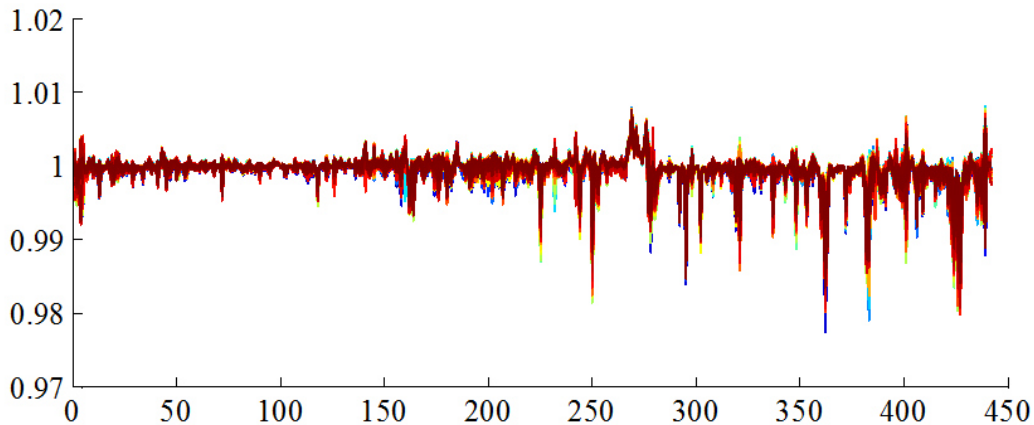
Abbildung 106: (n-0)-Spannungsbänder aller Knoten für alle Zeitpunkte des Szenarienjahrens
