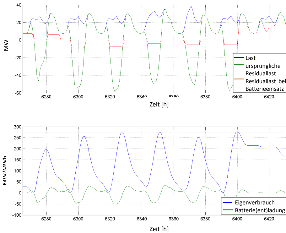
Abbildung 56: Beispiel eines berechneten Batterieeinsatzplanes für einen HÖS-Netznoten mit einer regionalen PV-Durchdringung in der Haushaltslast von 66 Prozent im Jahresdurchschnitt und einer zugehörigen Batteriekapazität von 276 MWh
