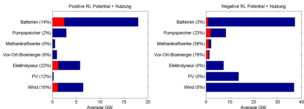
Abbildung 97: Simulierte Ausnutzung des vorhandenen Potenzials zur Regelleistungserbringung der verschiedenen Quellen für den Fall einer dynamischen Dimensionierung der vorzuhaltenden Regelleistung
