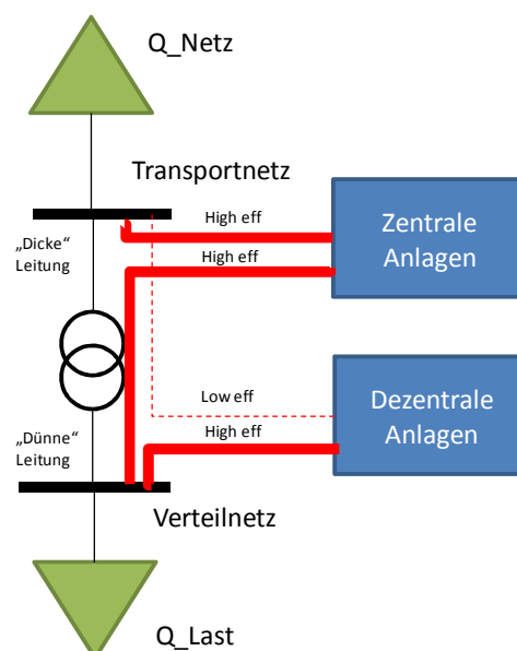
Abbildung 110: Schematische Darstellung der Blindleistungserbringung zentraler und dezentraler Stromerzeugers ins Transport- und Verteilungsnetz
