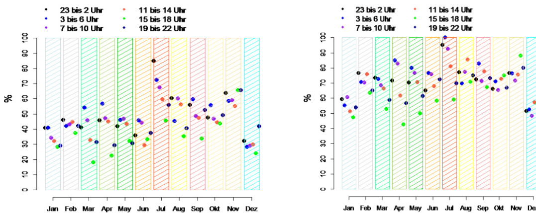
Abbildung 81: a) Differenzen zwischen Beobachtung und Prognose (angegeben in Prozent der Nennleistung), die kleiner als 5 Prozent sind. b) Differenzen zwischen Beobachtung und Prognose (angegeben in Prozent der Nennleistung), die kleiner als 10 Prozent sind (jeweils Windpark 3 – Prognosejahr 2011)
