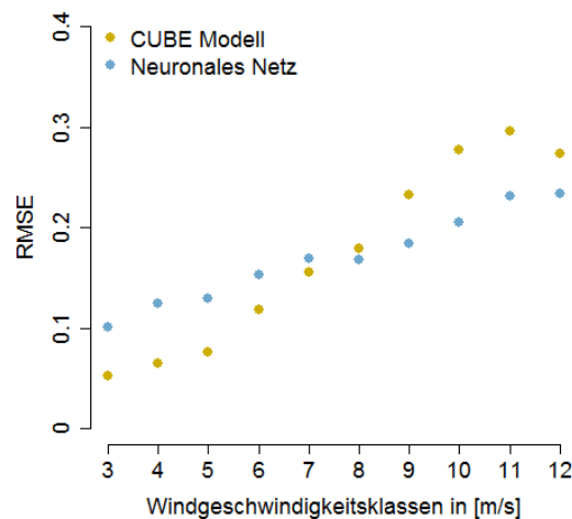
Abbildung 86: Windklassenspezifischer RMSE für Park 4
