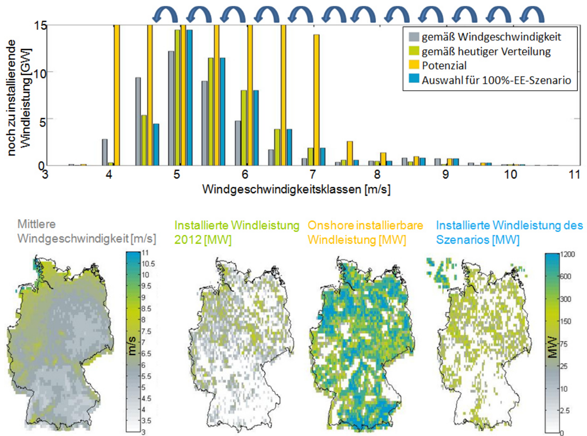
Abbildung 12: Erstellung des Onshore-Windenergie-Szenarios
