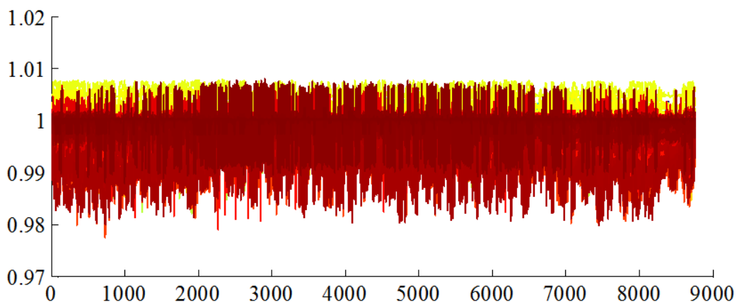
Abbildung 107: (n-0)-Spannungsbänder aller Stunden des Szenarienjahrens von allen Knoten
