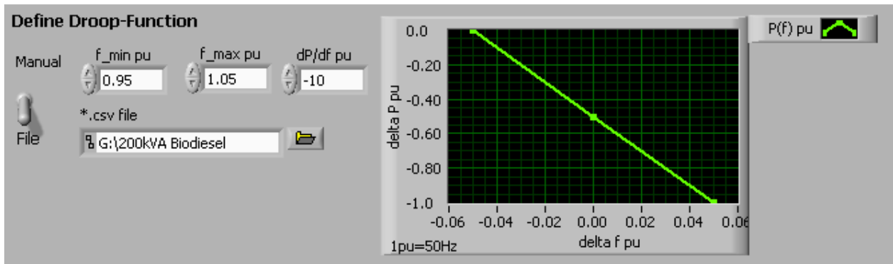
Abbildung 131: Angesetzte \Delta P/\Delta f -Statik der Windenergieanlage
