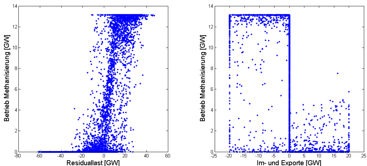
Abbildung 51: a) Simulierter Zusammenhang zwischen Methanisierung und Residuallast (links) bzw. b) Leistungsimpport und -export (rechts) für jede Stunde des Szenariensjahres und für ganz Deutschland
