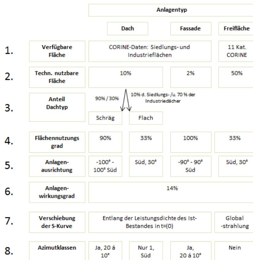
Abbildung 22: Flächenberechnung PV
