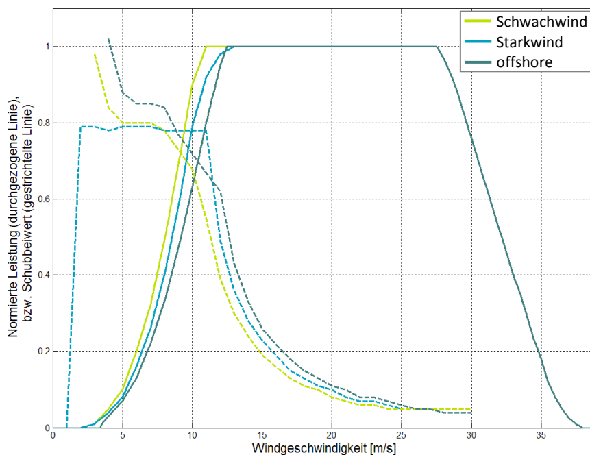
Abbildung 17: Leistungs- und Schubbeiwert-Kennlinien der Windenergieanlagen im Szenario
