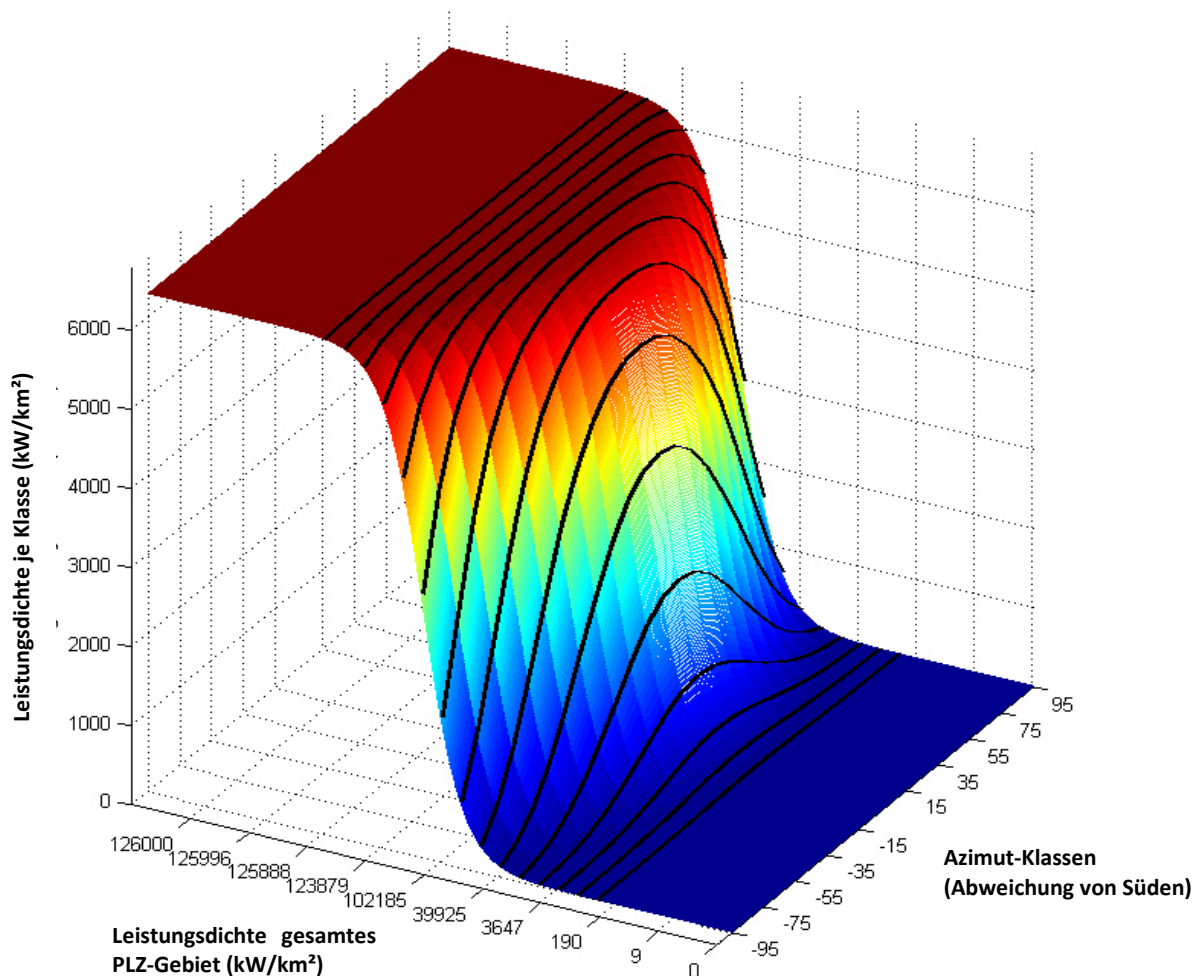
Abbildung 24: Verteilungskurven der Leistungsdichte für unterschiedliche Ausbauzustände und Ausrichtungen der PV-Schrägdachanlagen eines PLZ-Gebietes
