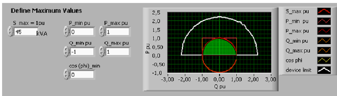
Abbildung 127: Angesetztes P/Q-Diagramm der Biogasanlage
